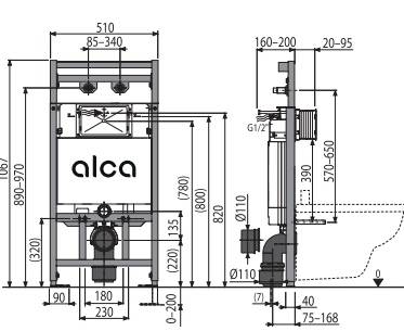
A108F/1100 Montážní rám s nádržkou pro výlevku s odpadem DN90/110 a baterii
