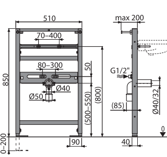
A104/850 Montážní rám pro umyvadlo
