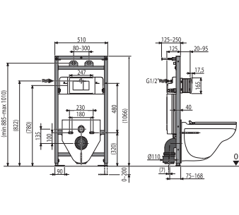
A108F 5:1 SET Set montážního rámu, výlevky, izolační desky, mřížky a ovládacího tlačítka
