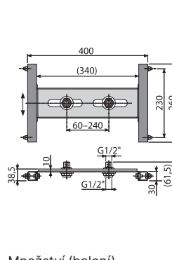
A117B Montážní rám do sádkartonové konstrukce pro baterii
