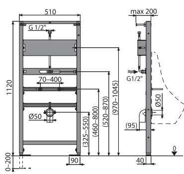
A107S/1120 Montážní rám pro pisoár a senzor
