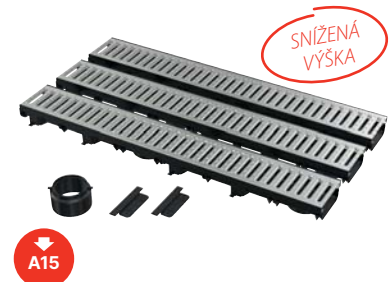
AVZ112-G102 Garážový set 3 m (2x čelo, 1x hrdlo DN110)
