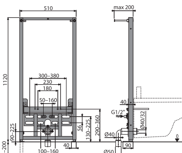
A105/1120 Montážní rám pro bidet
