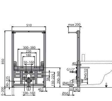
A105/850 Montážní rám pro bidet
