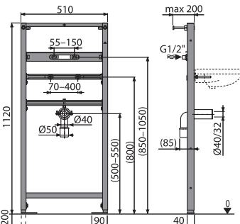
A104A/1120 Montážní rám pro umyvadlo a baterii
