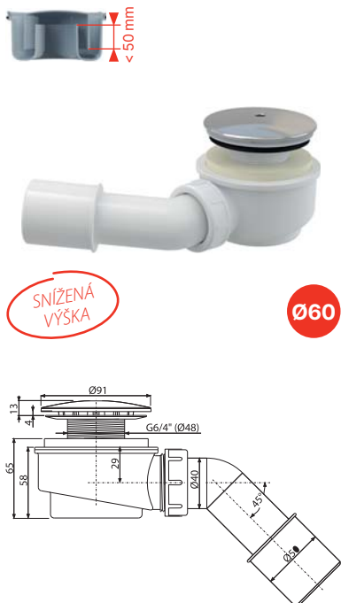
A471CR-60 Odtoková souprava vaničková, chrom
