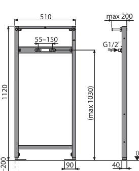
A104B/1120 Montážní rám pro baterii
