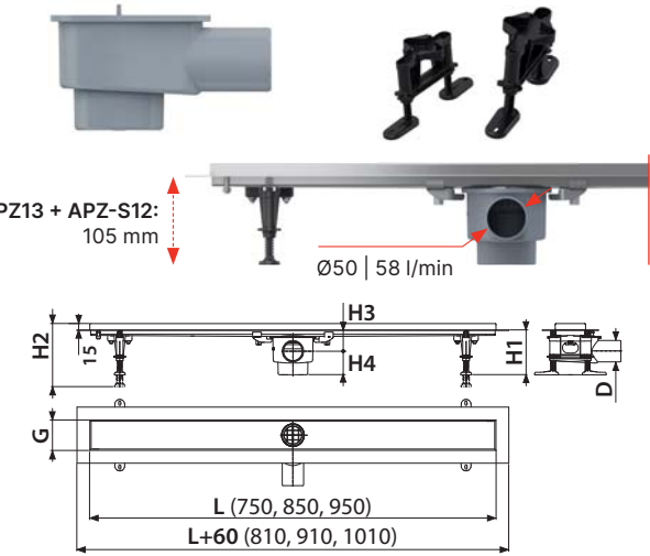
APZ-S12 Sifon DN50 a sada nastavitelných noh
