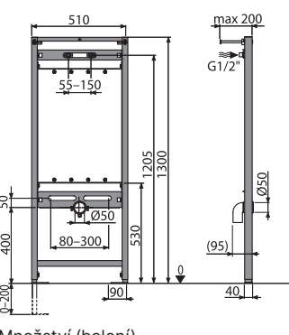
A108/1300 Montážní rám pro výlevku a baterii
