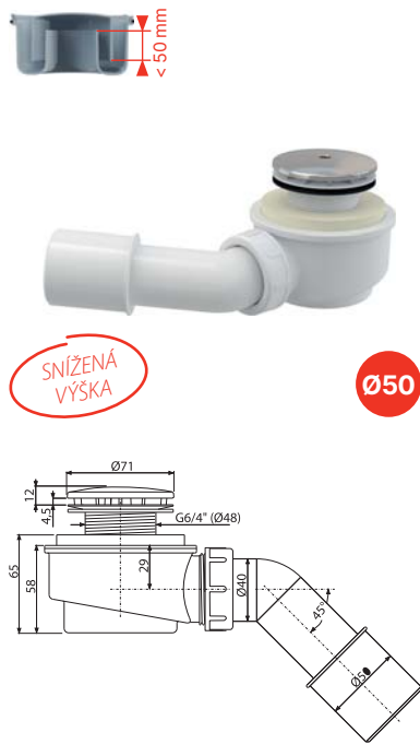
A471CR-50 Odtoková souprava vaničková, chrom
