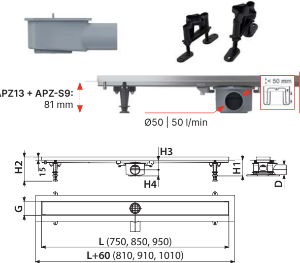
APZ-S9 Nízký sifon DN50 a sada nastavitelných noh
