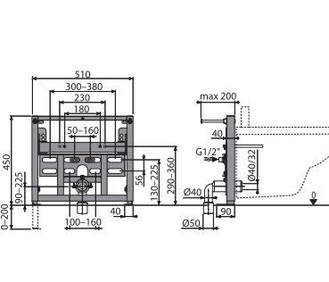
A105/450 Montážní rám pro bidet
