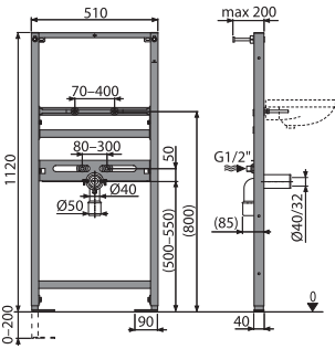
A104/1120 Montážní rám pro umyvadlo
