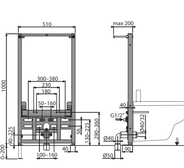
A105/1000 Montážní rám pro bidet
