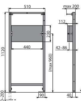
A104PB/1120 Montážní rám pro podomítkovou baterii
