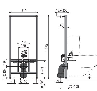
A114/1120 Montážní rám pro závěsné WC
