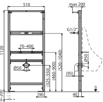
A107/1120 Montážní rám pro pisoár
