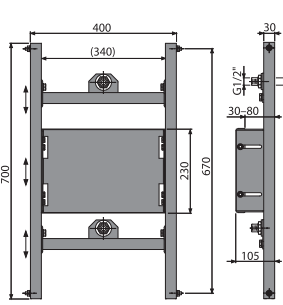
A117PB Montážní rám do sádkartonové konstrukce pro podomítkovou baterii
