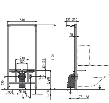
A113/1120 Montážní rám pro závěsné WC kombi
