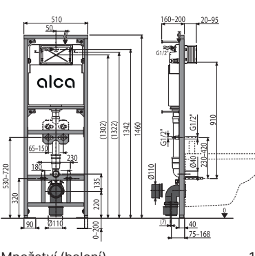
A108F/1500 Montážní rám s nádržkou pro výlevku s odpadem DN90/110 a baterii
