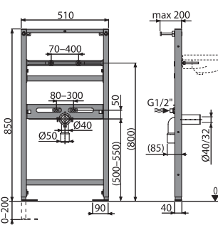
A104/1000 Montážní rám pro umyvadlo
