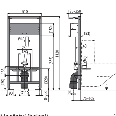
A114S/1120 Montážní rám pro závěsné WC a senzor
