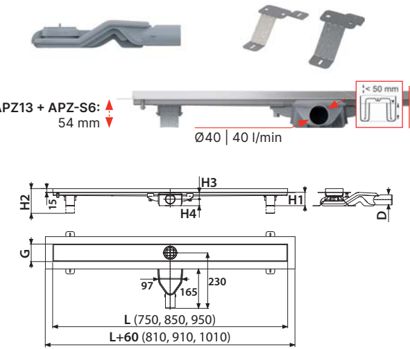
APZ-S6 Extra-nízký sifon DN40 a sada nastavitelných noh
