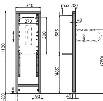
A106/1120 Montážní rám pro madlo
