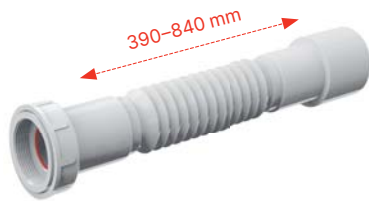
A793 Flexi připojení 6/4" s redukcí na 5/4"×50/40 plast
