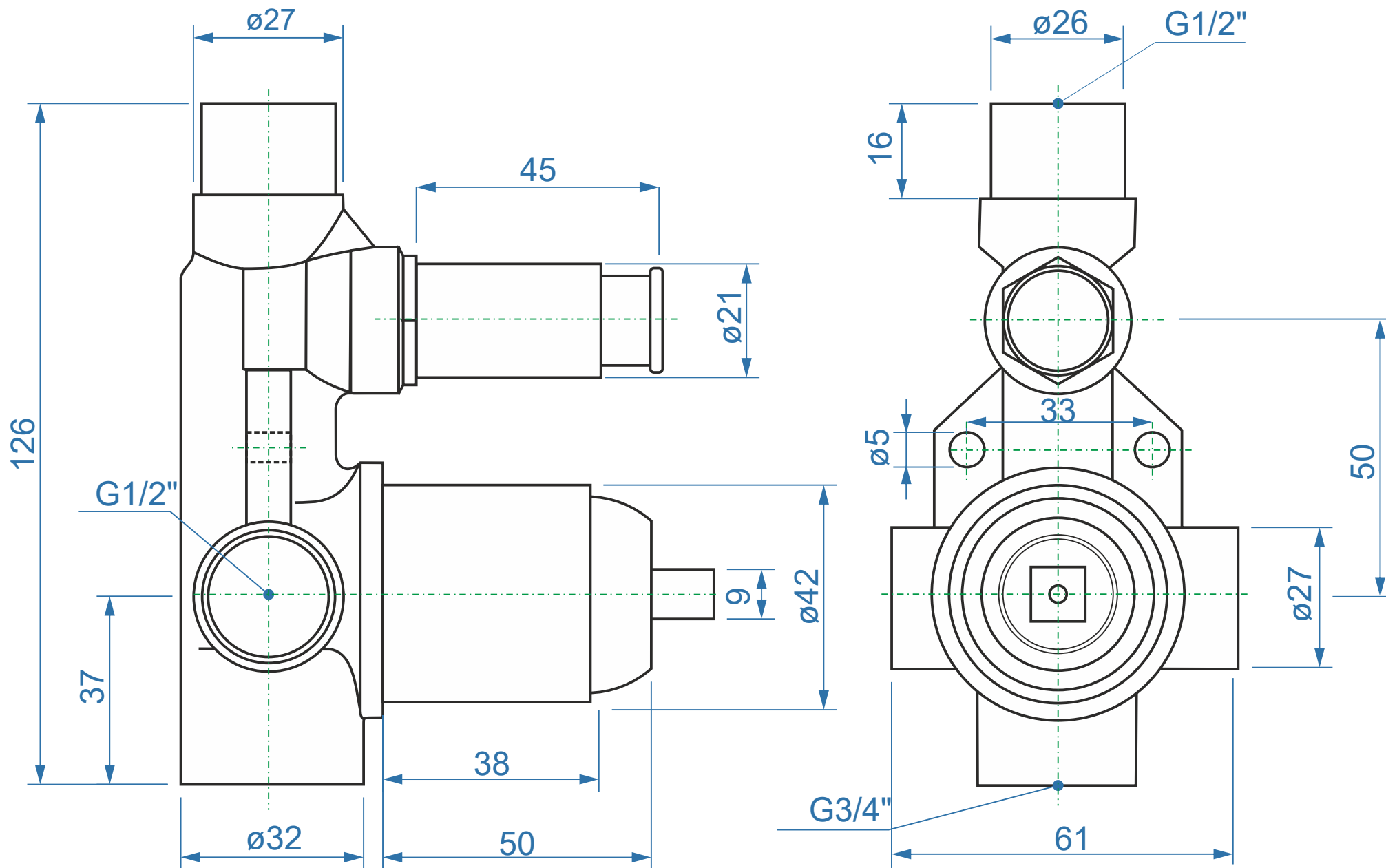
AQ-BOX-066-35 tělo baterie
